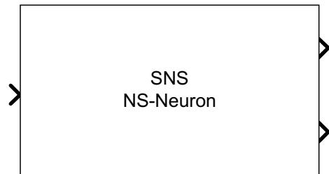
NonSpikingNeuron
