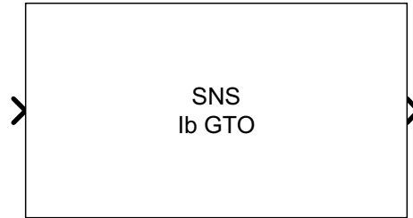
IbGolgiTendon
