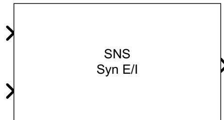
NonSpikingSynapse
