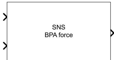
BPAForce
