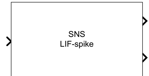
SpikingLIFNeuron
